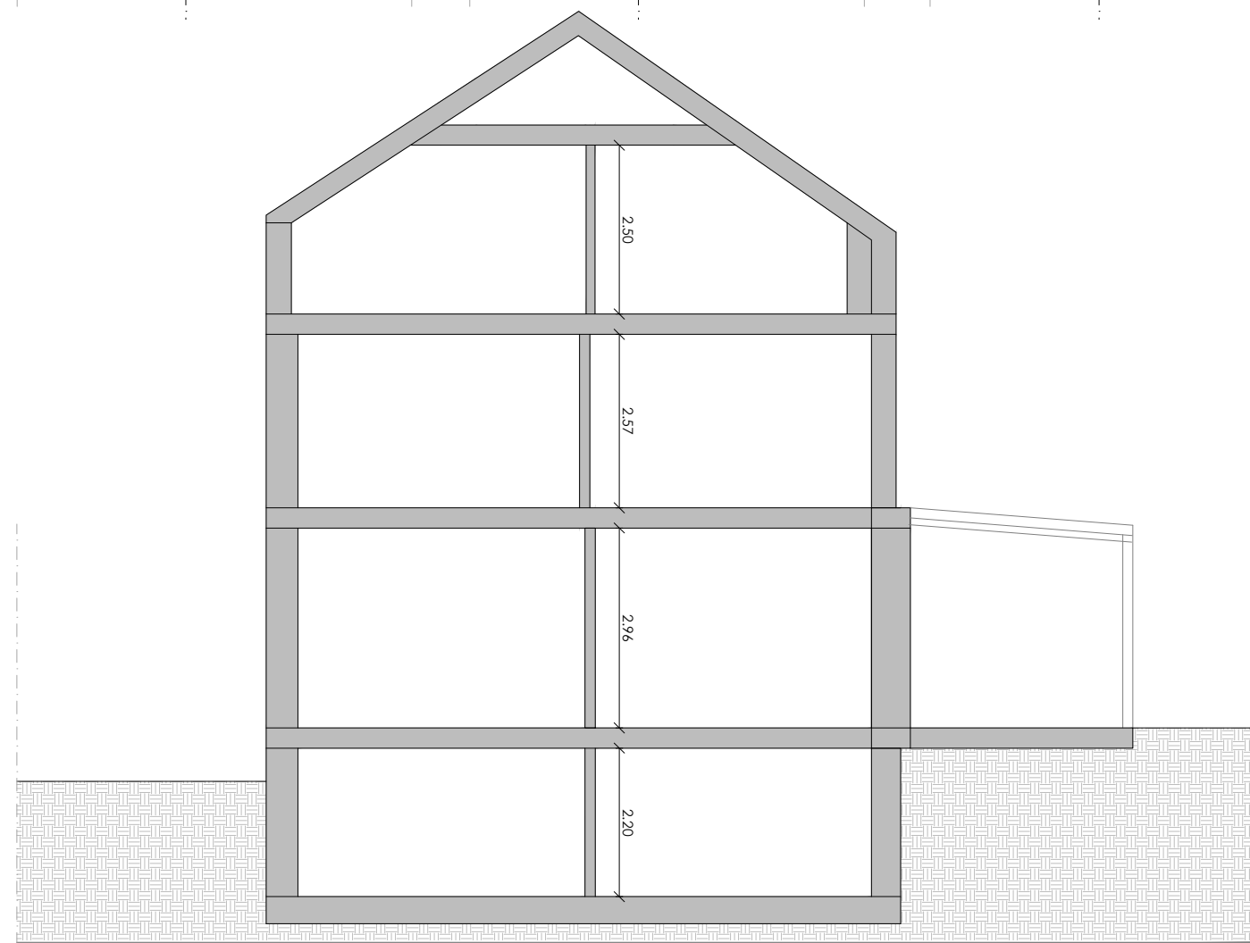
COUPE A-A'
