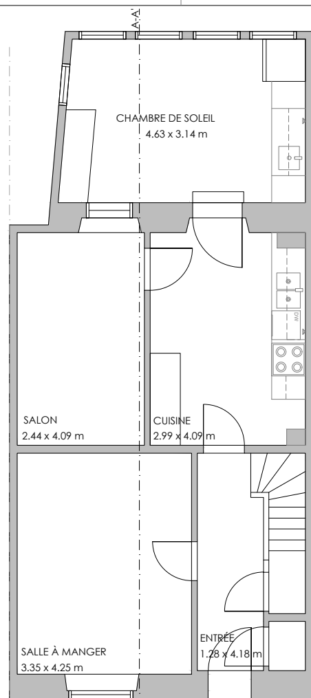
REZ-DE-CHAUSSÉE
