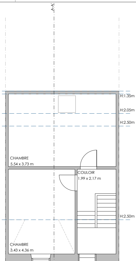
2EME ÉTAGE
