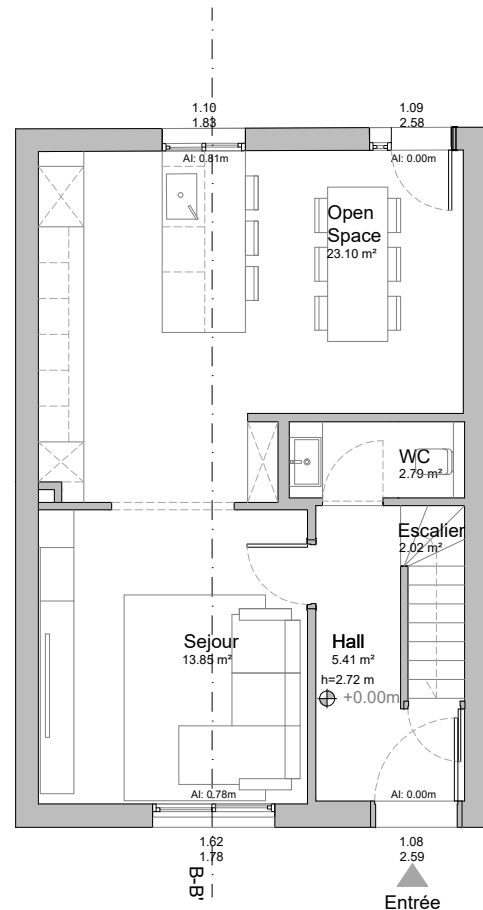
PLAN RDC
