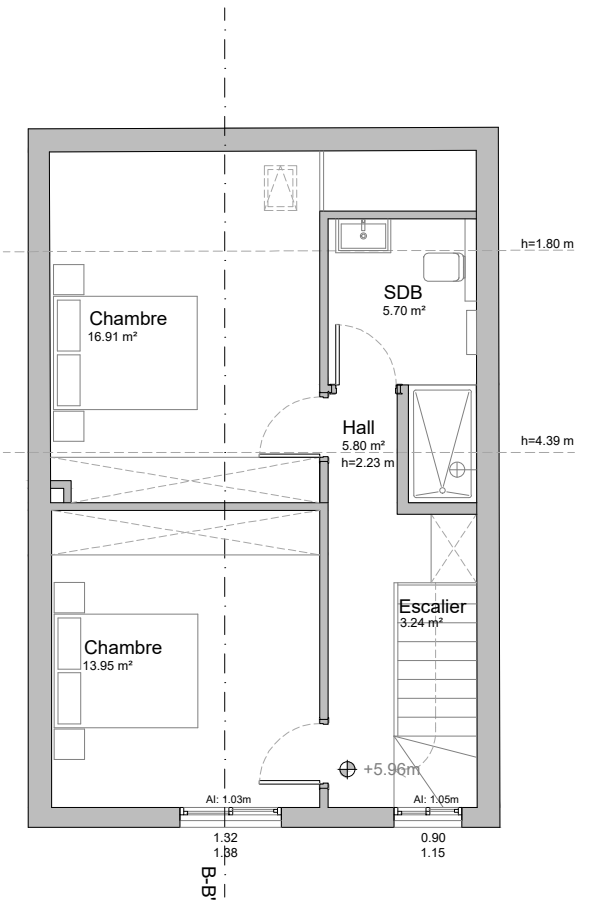
PLAN ETAGE 2
