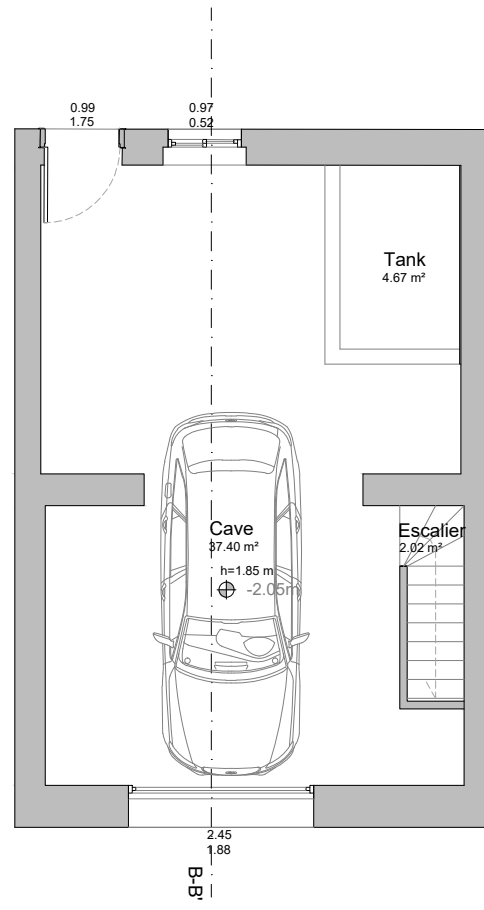
PLAN SOUS-SOL
