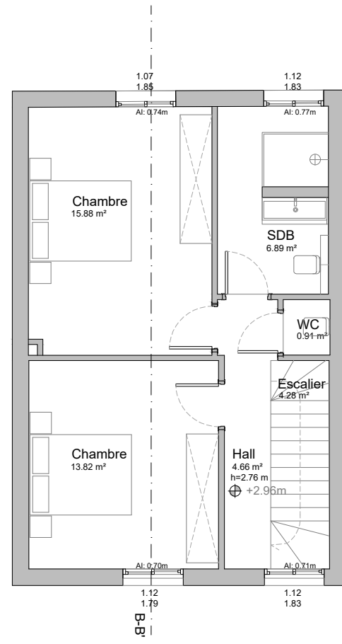
PLAN ETAGE 1
